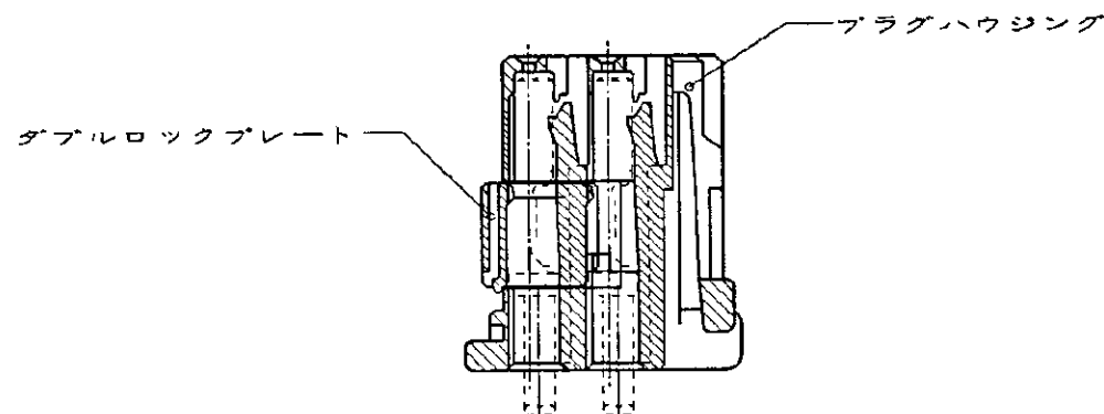
断面 A-A (SECT. A-A)
